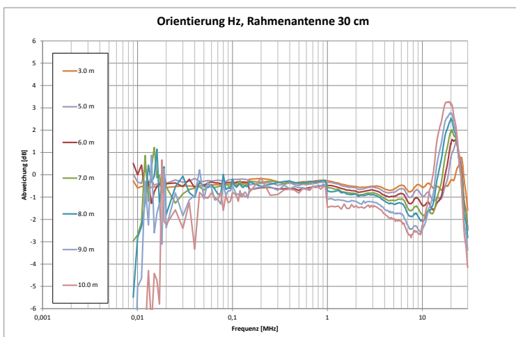
Bild 14: NSA Messung in H_z Orientierung in verschiedenen Messabständen von 3 bis 10 m (ohne 4 m Messabstand); Rahmenantennen 30 cm
