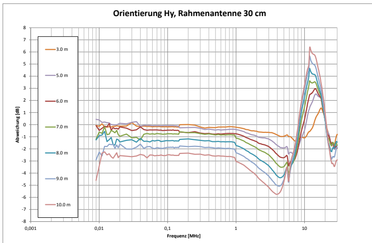
Bild 13: NSA Messung in H_y Orientierung in verschiedenen Messabständen von 3 bis 10 m (ohne 4 m Messabstand); Rahmenantennen 30 cm
