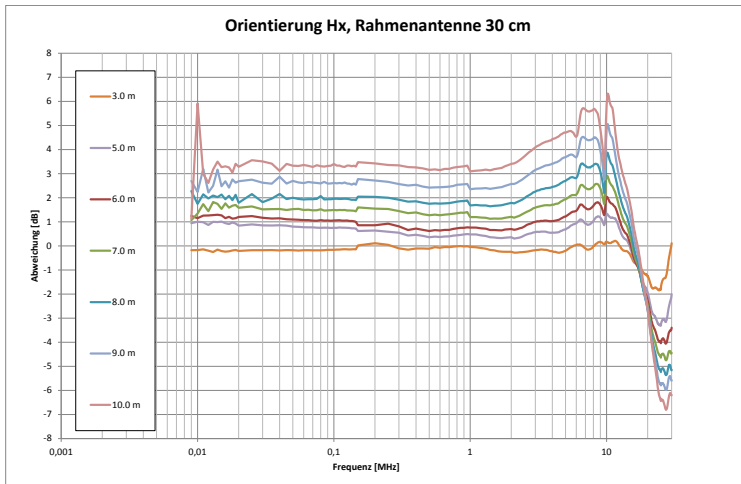
Bild 12: NSA Messung in H_x Orientierung in verschiedenen Messabständen von 3 bis 10 m (ohne 4 m Messabstand); Rahmenantennen 30 cm
