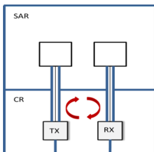
Bild 3: Kopplungseffekt bei Standardaufbau
