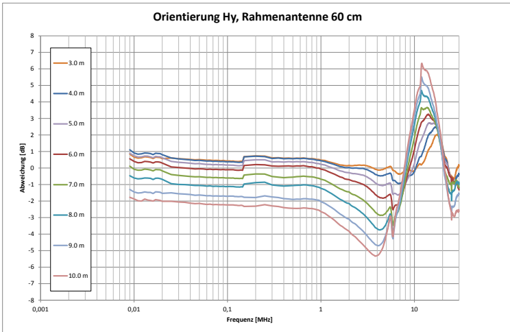
Bild 10: NSA Messung in H_y Orientierung in verschiedenen Messabständen von 3 bis 10 m; Rahmenantennen 60 cm
