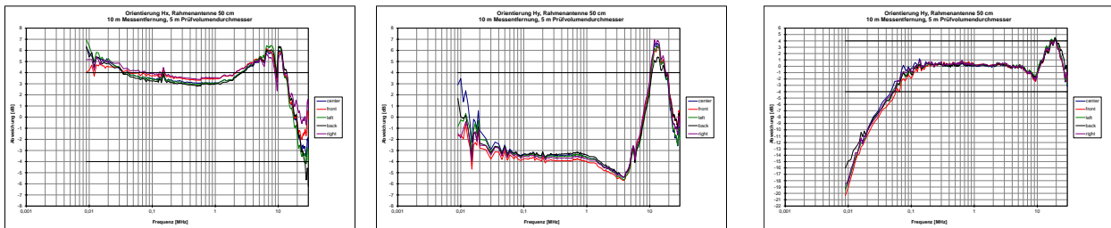
Bild 18: NSA Messung (2012) in den Orientierungen H_x , H_y und H_z in 10 m Messabstand; Rahmenantennen 50 cm Durchmesser
