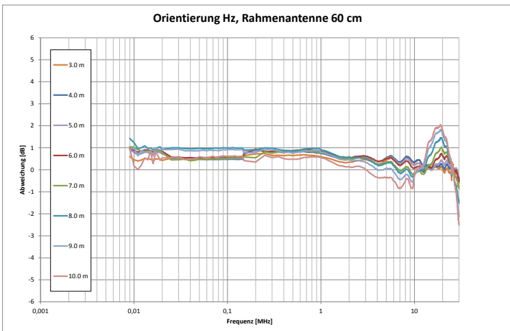
Bild 11: NSA Messung in H_z Orientierung in verschiedenen Messabständen von 3 bis 10 m; Rahmenantennen 60 cm
