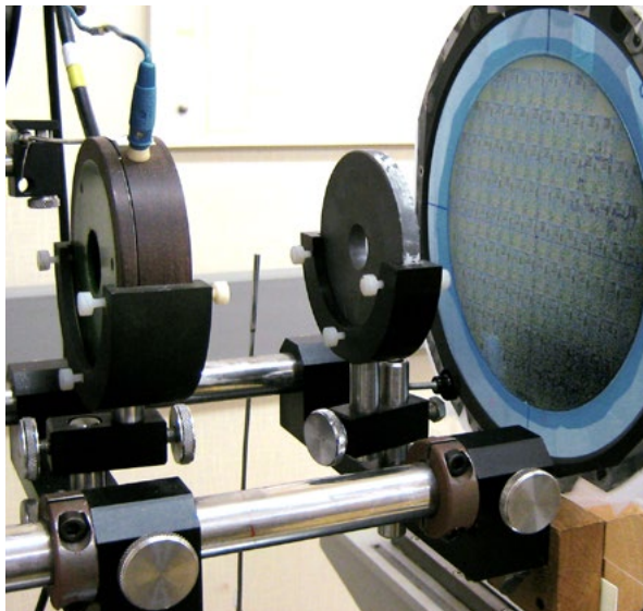
Silizium-Wafer-Röntgenbestrahlungstest
